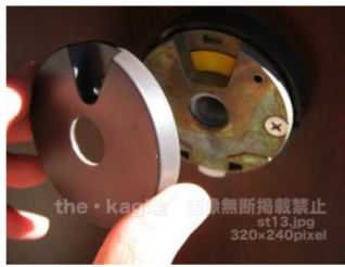
15.こちらの2本のビスを緩めて取り外しましょう。
