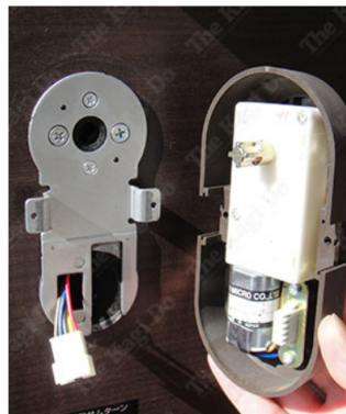
12. 下部シリンダーを外していきます。上部シリンダーと同様【手順4】～【手順9】まで行います。
