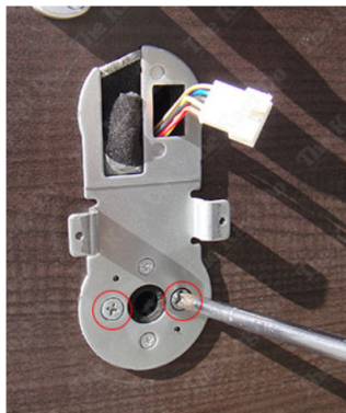
10. 赤丸部分のシリンダーの2か所の固定ネジをプラスドライバーで外します。赤丸部分のネジはそのまま大丈夫です。
